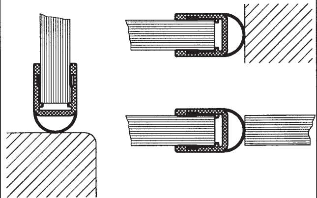
Art.Nr.: 6906 Hartweich-Lippendichtung
