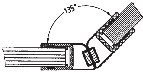
Art.Nr.: 6900 Magnetprofil 135°
