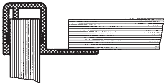
Art.Nr.: 6904 Eckanschlagprofil
